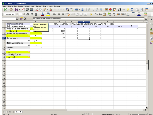
Рис. 3: Шаблон для численного решения четырехшаговым методом Адамса–Башфорта обыкновенных дифференциальных уравнений второго порядка
