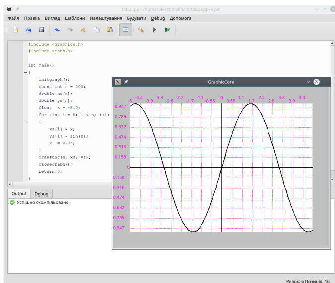
Рис. 1: Оболочка Kuzya
