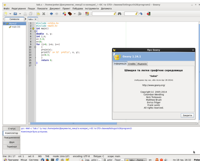
Рис. 2: Оболочка Geany
