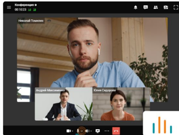
Шумоподавление
