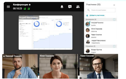
Автогенерация раскладки
