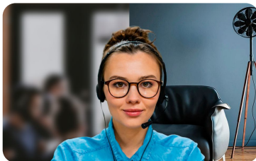
Виртуальный фон
