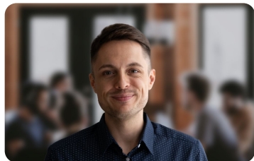
Размытие фона
